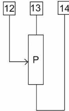
Potentiomètre de recopie 0,1 - 1 - 5 - 10 KOhm
